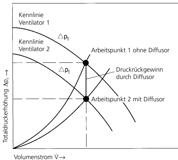
Bild 2: Druckrückgewinnung
