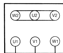
Połączenie w gwiazdę (wysokie napięcie)
