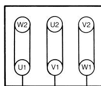
Połączenie w trójkąt (niskie napięcie)
